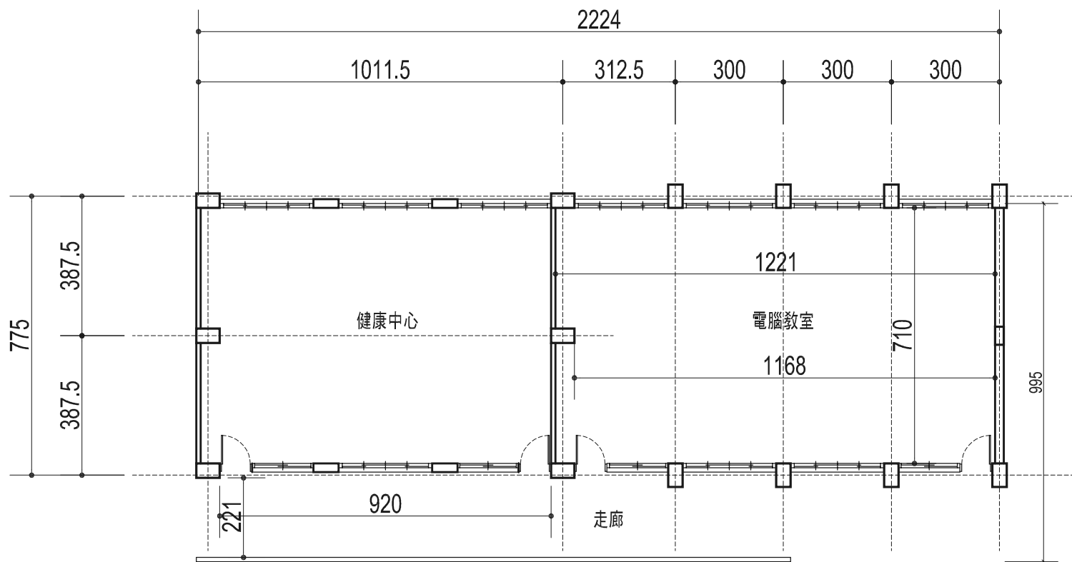
二樓平面圖
