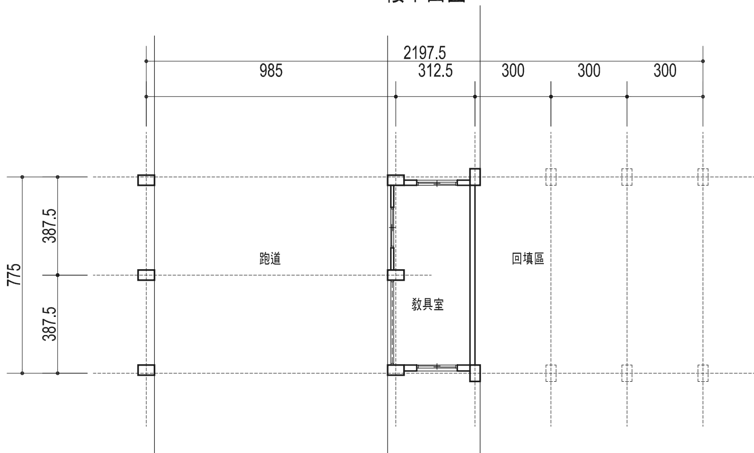
一樓平面圖
