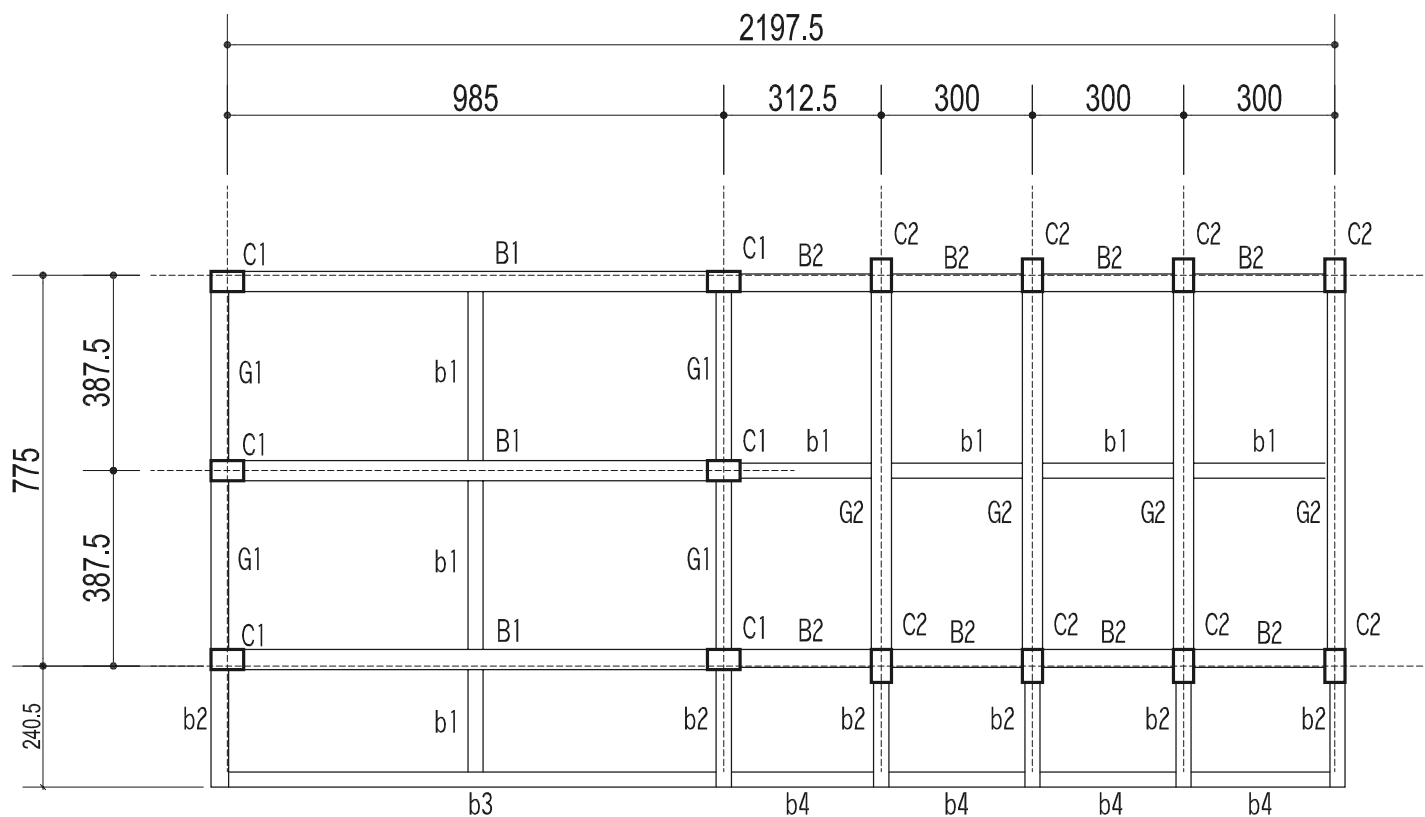
屋頂結構平面圖
