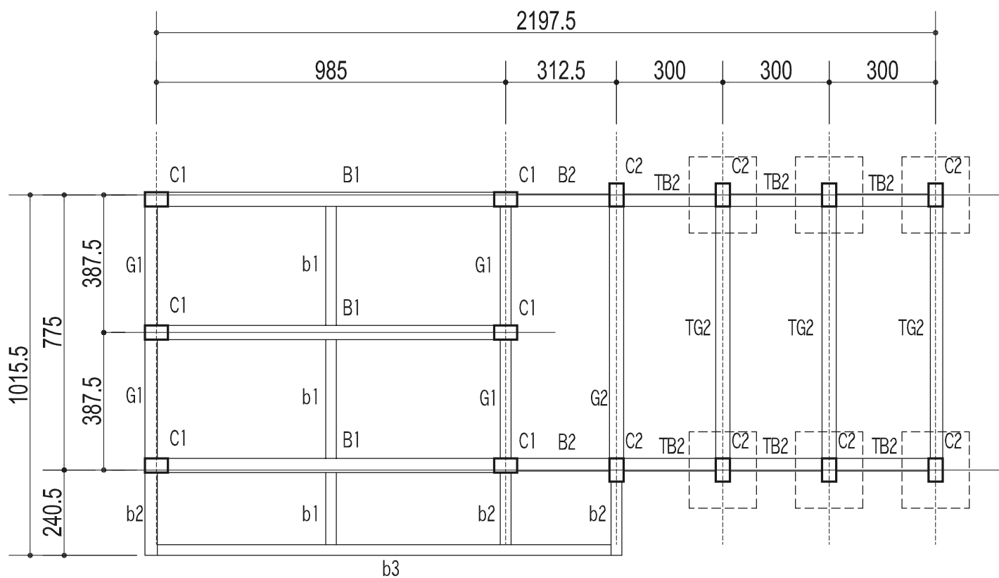
二樓結構平面圖
